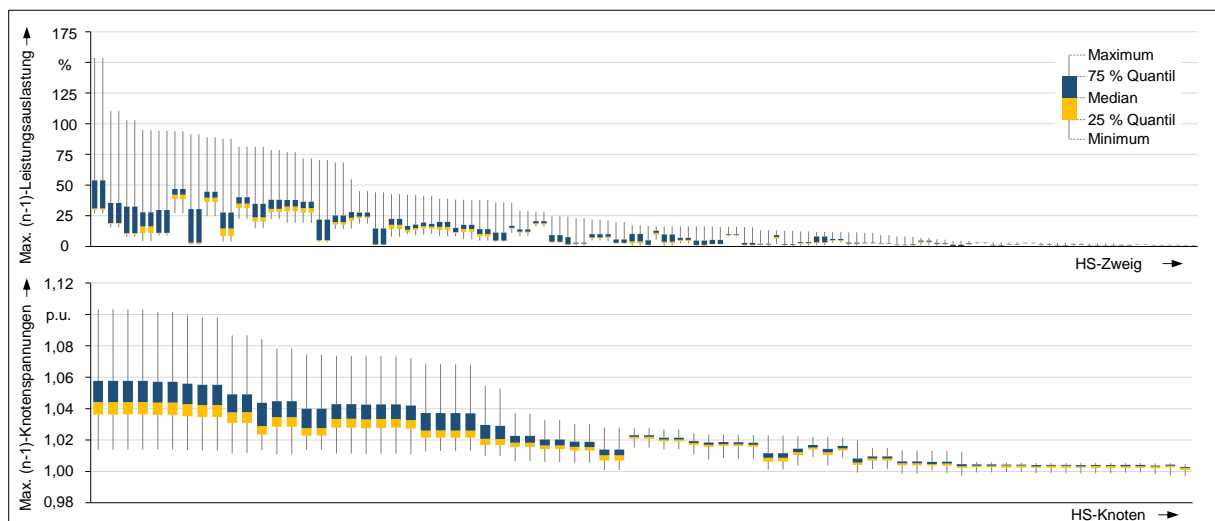
Abbildung 4: Maximale (n-1) -Leitungsauslastungen und (n-1) -Knotenspannungen des HS-Netzes bei vollständiger Modellierung der HöS-Ebene (Quantile bezogen auf Stunden des Jahres)
