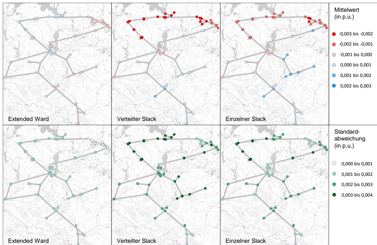
Abbildung 8: Mittelwert und Standardabweichung des Modellierungsfehlers der (n-1)-Knotenspannungen bei vereinfachter Modellierung der HöS-Ebene
