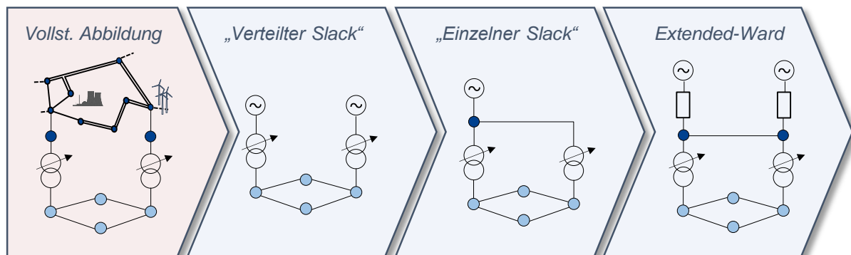
Abbildung 2: Übersicht der untersuchten Modelle zur Abbildung des HöS-Netzes
