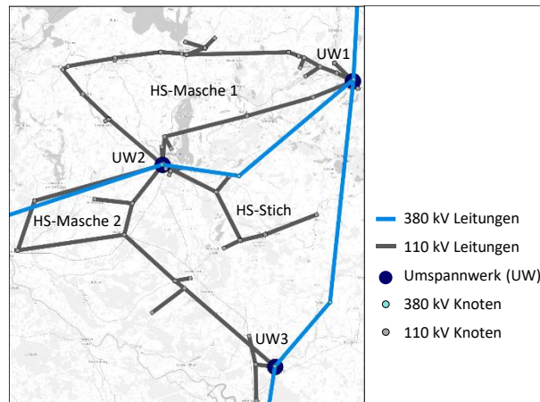
Abbildung 3: Betrachteter Ausschnitt des vollständigen HöS/HS-Netzmodells
