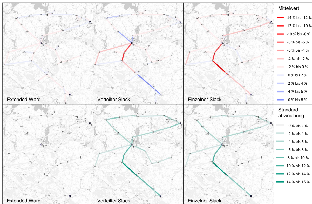
Abbildung 6: Mittelwert und Standardabweichung des Modellierungsfehlers der (n-1)-Leitungsauslastungen bei vereinfachter Modellierung des HöS-Netzes
