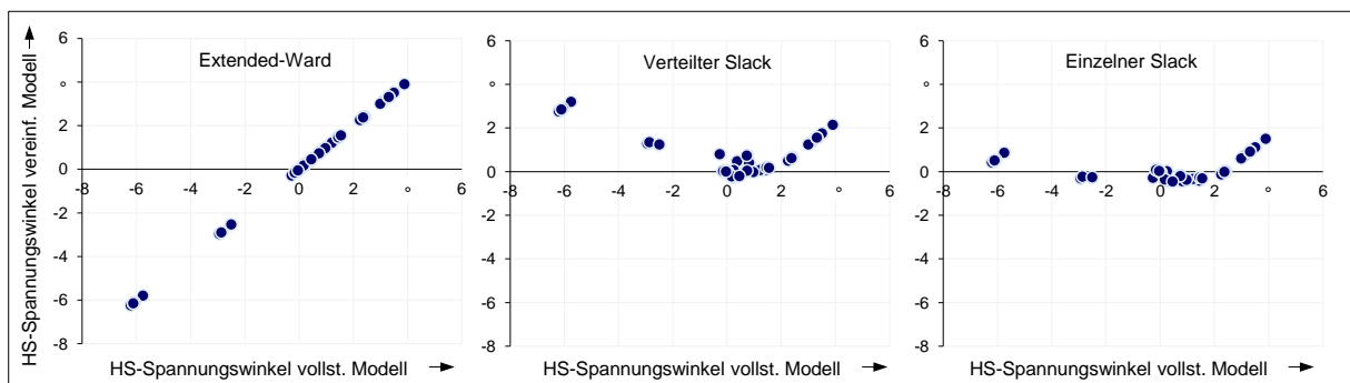
Abbildung 7: Vergleich der HS-Spannungswinkel zwischen vollständigem und vereinfachtem HöS-Netzmodell für eine exemplarische Stunde mit hohem Transportbedarf im Übertragungsnetz
