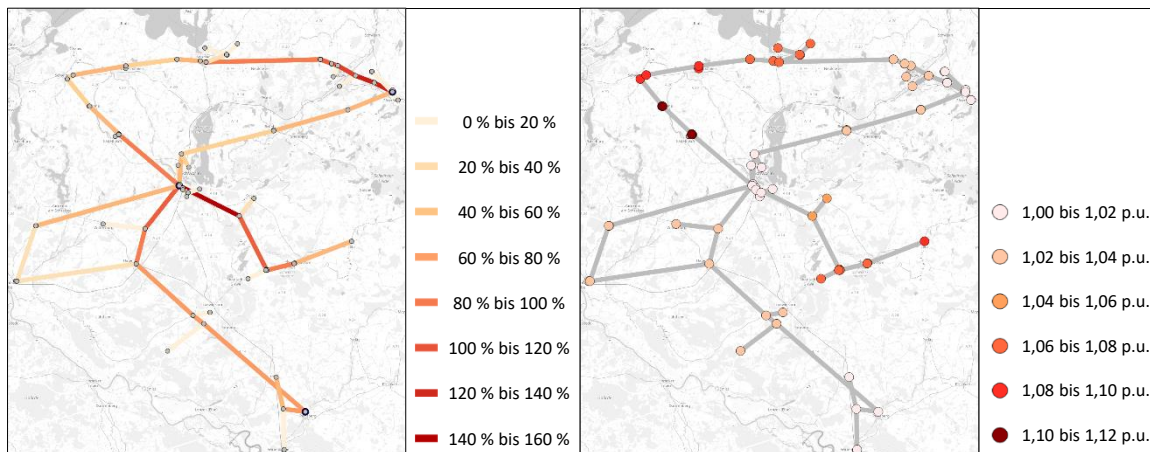
Abbildung 5: Maximale (n-1)-Leitungsauslastungen und (n-1)-Spannungen der Jahressimulation
